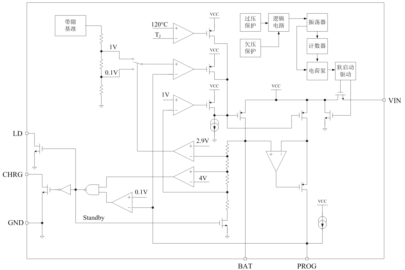
图 2: QX4059 的内部电路方框图
