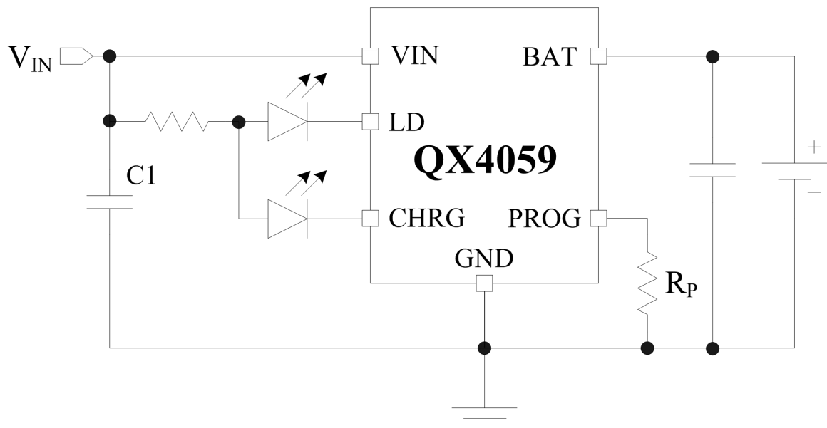
图 1 : QX4059 典型应用电路图
