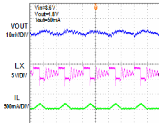
PFM MODE
