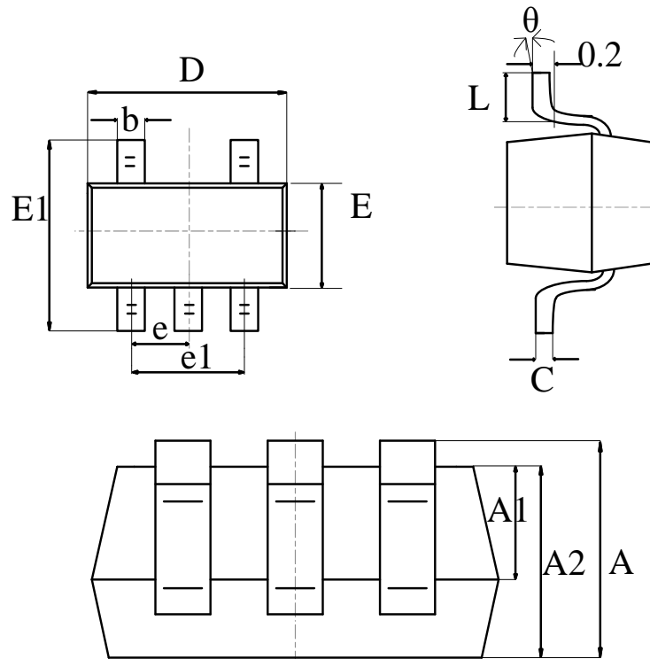
SOT23-5
